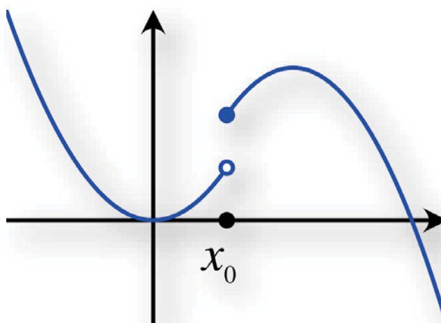
نمودار یک تابع چند ضابطه ای
